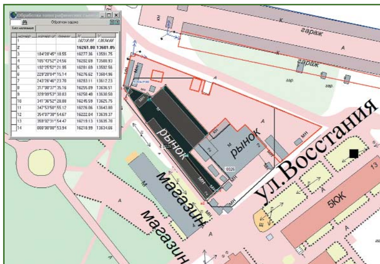
Рис. 4 Пример обработки результатов тахеометрической съемки в ПО «Геомастер»
